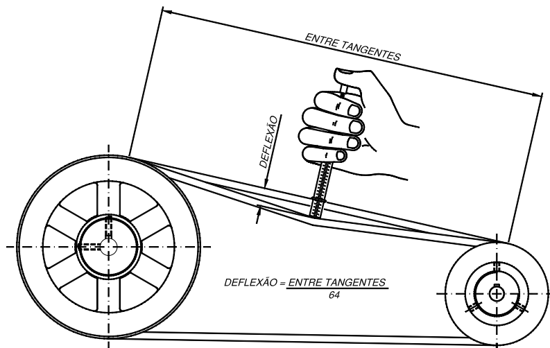
Fig. 07 - Ajuste da tensão da correia
