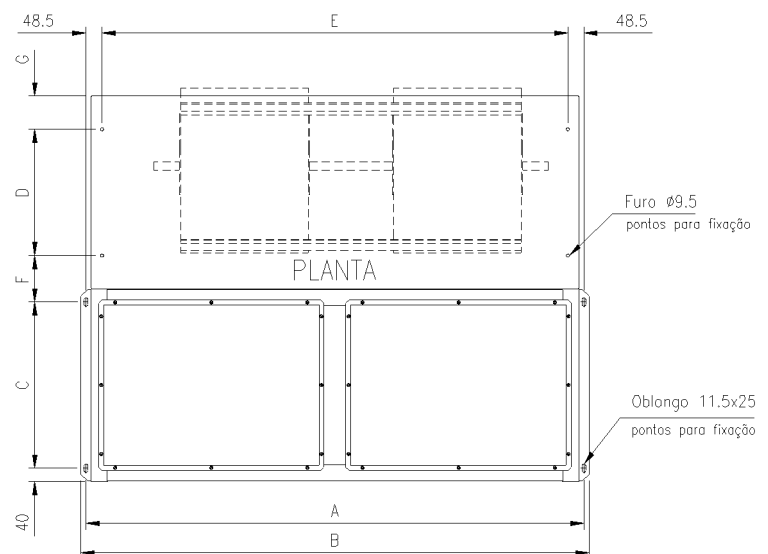
Fig. 25 - Montagem dos Módulos Ventilador e Serpentina CXPA 050 a 500 - Horizontal - Vista Superior
