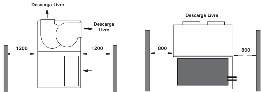
Fig. 28 - Espaços sugeridos para manutenção e circulação de ar para os módulos serpentina e ventilador. (Gabinete Vertical)
