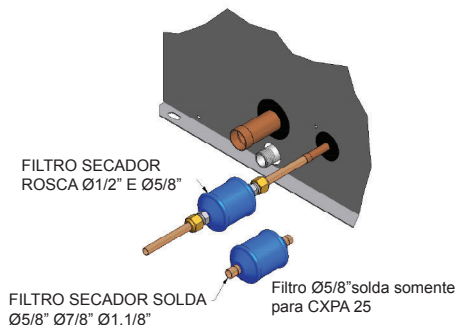
ESQUEMA DE MONTAGEM FILTRO SECADOR
