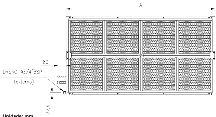
Fig. 18 - Dimensional Módulo Serpentina 200 a 300
