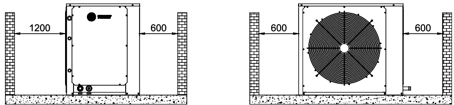
Fig. 43 - Espaços sugeridos TRAE 200 a 250 - Descarga Vertical
