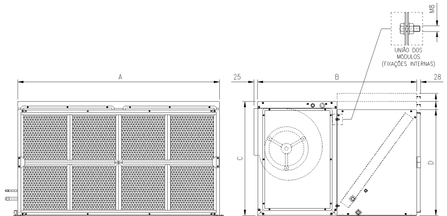
Fig. 24 - Montagem dos Módulos Ventilador e Serpentina CXPA 050 a 500 - Horizontal
